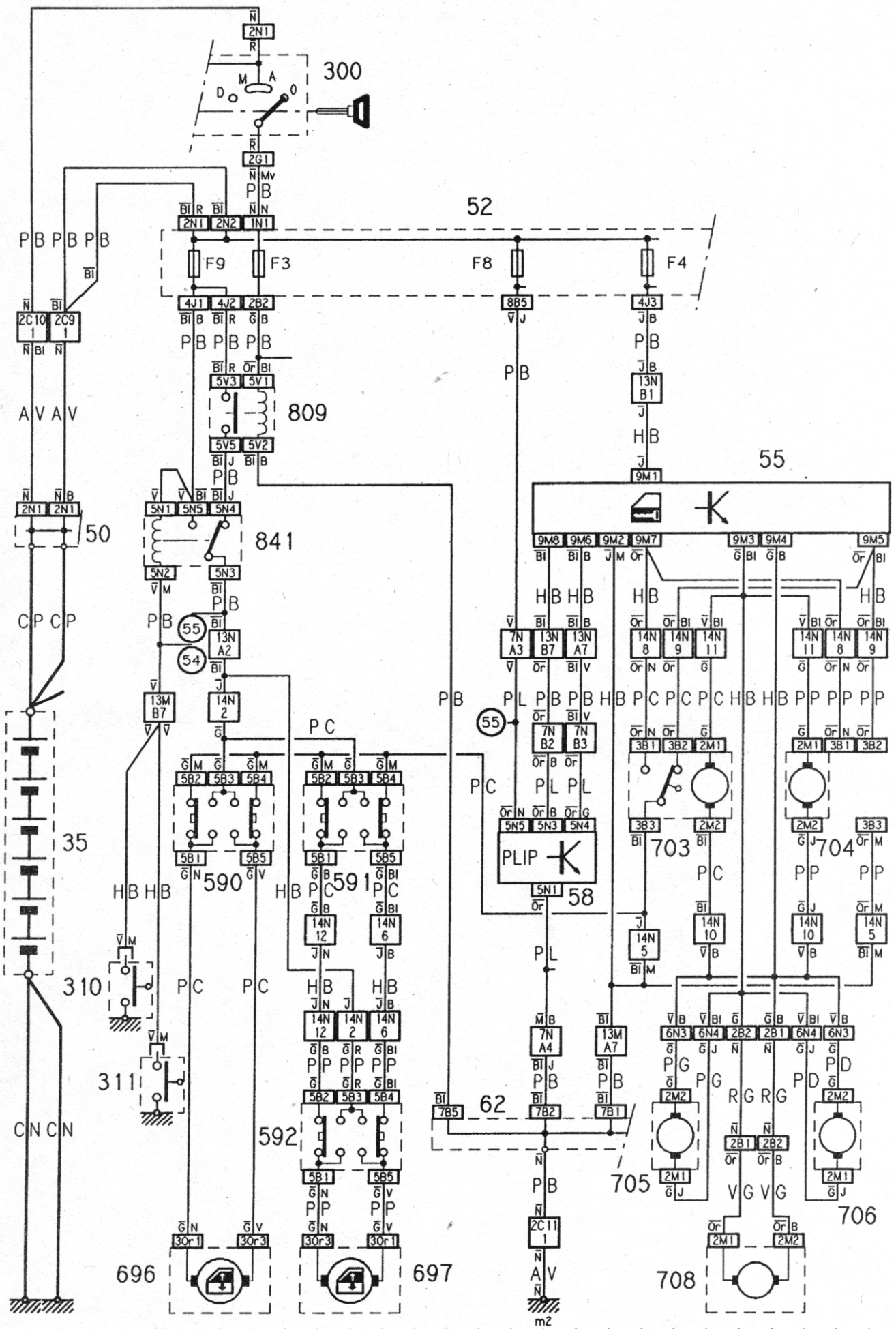
Lève-vitres électriques et condamnation centrale - circuit type
