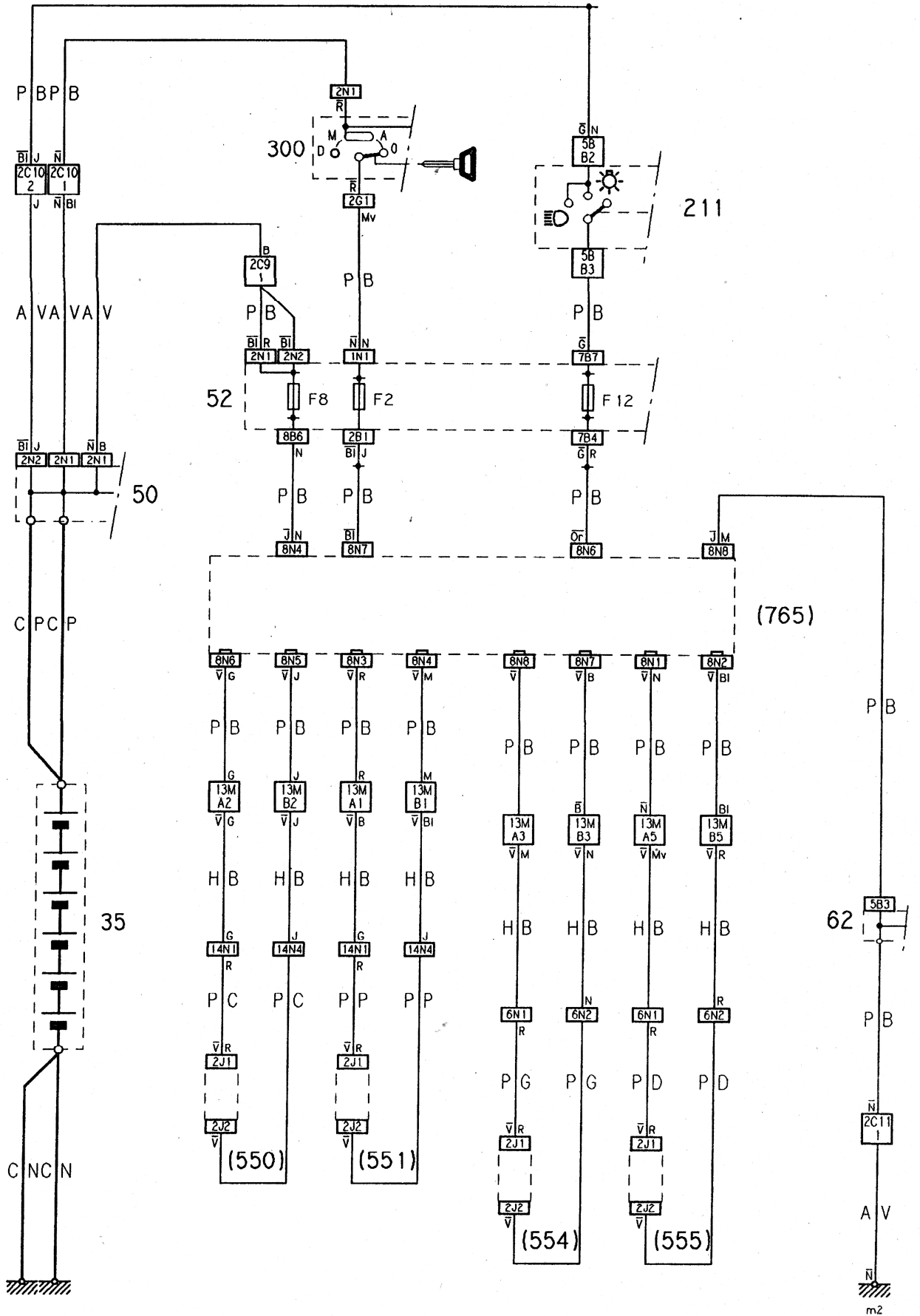
Autoradio (type à quatre haut-parleurs) - circuit type
