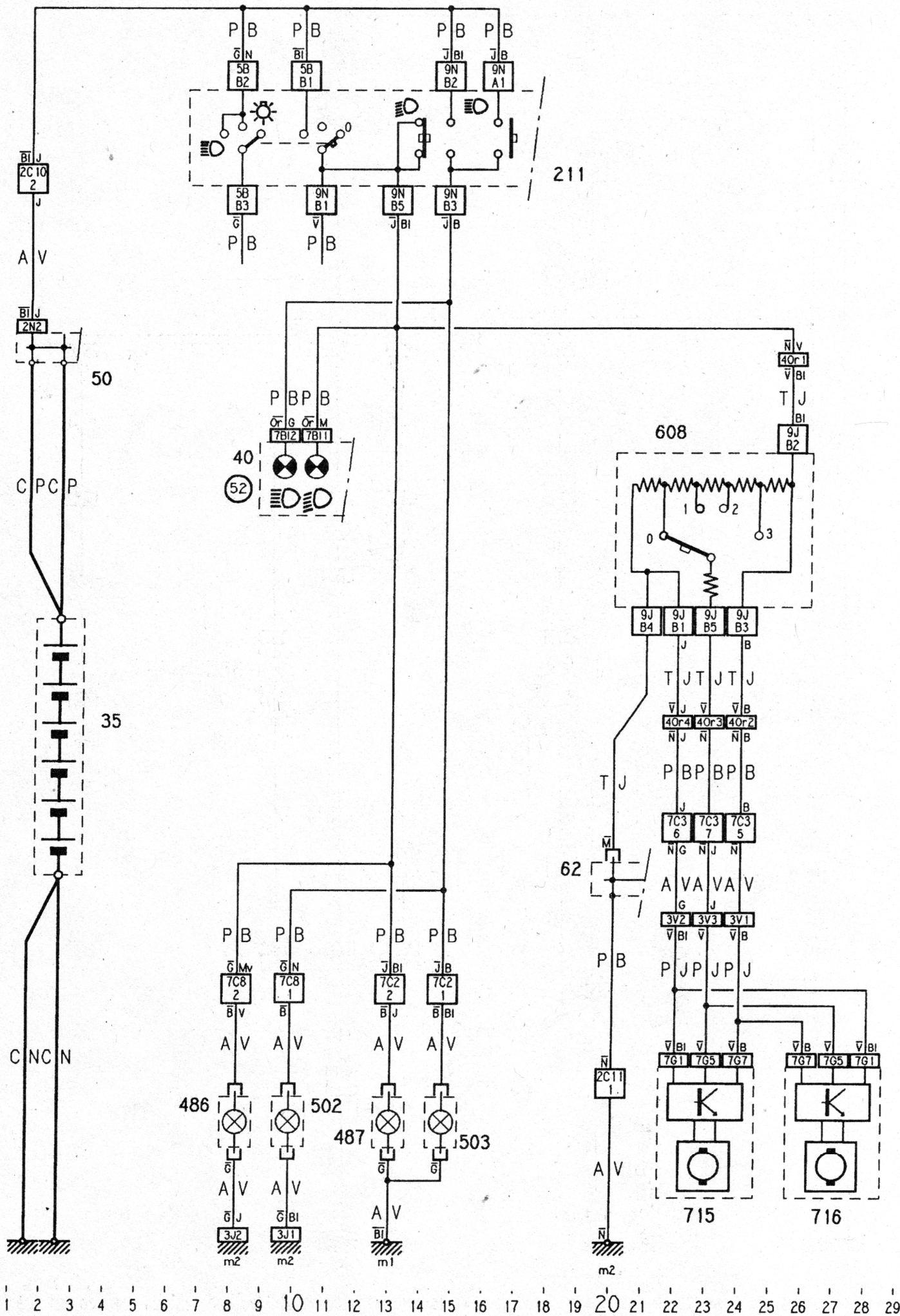
Réglage des projecteurs - circuit type
